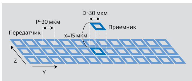
Рис.4. Реализация многоканальной индуктивной связи
