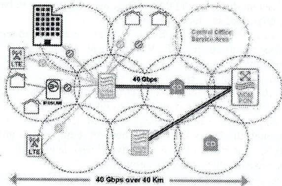
Fig. 2. Distribution units WDM-PON
