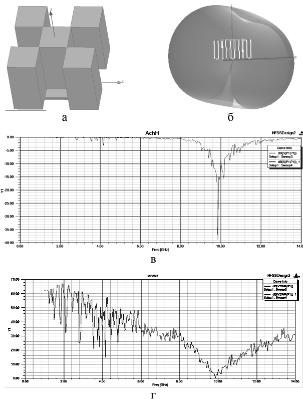
Рис. 2. Перший варіант квазіфрактальної DRA: а – схема живлення; б – ДС; в – АЧХ; г – VSWR
