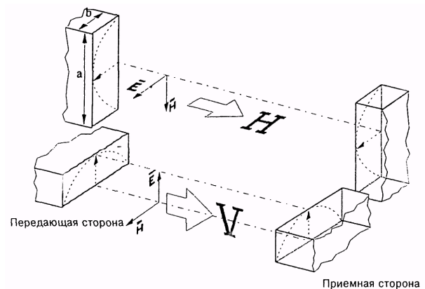
Рис. 1. Схема приема
